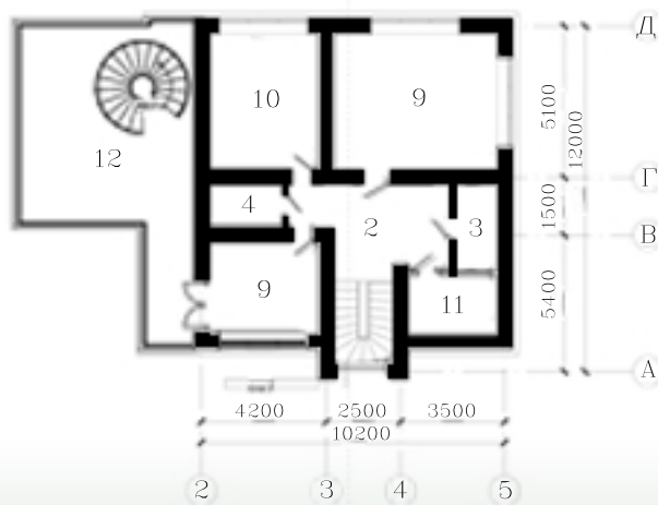
План Второго этажа М 1:100
