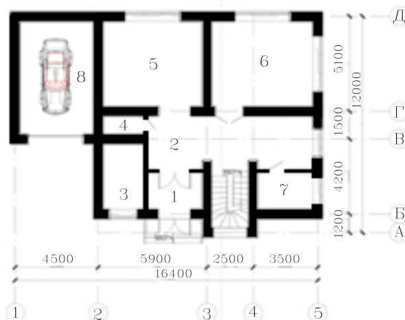
План первого этажа М 1:100
