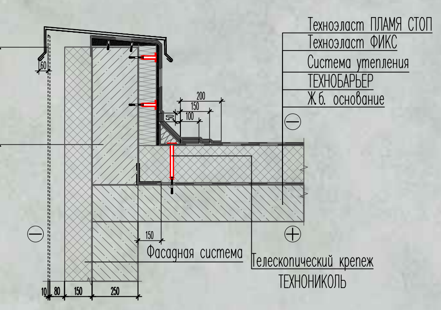
УЗЕЛ А, М 1:20
