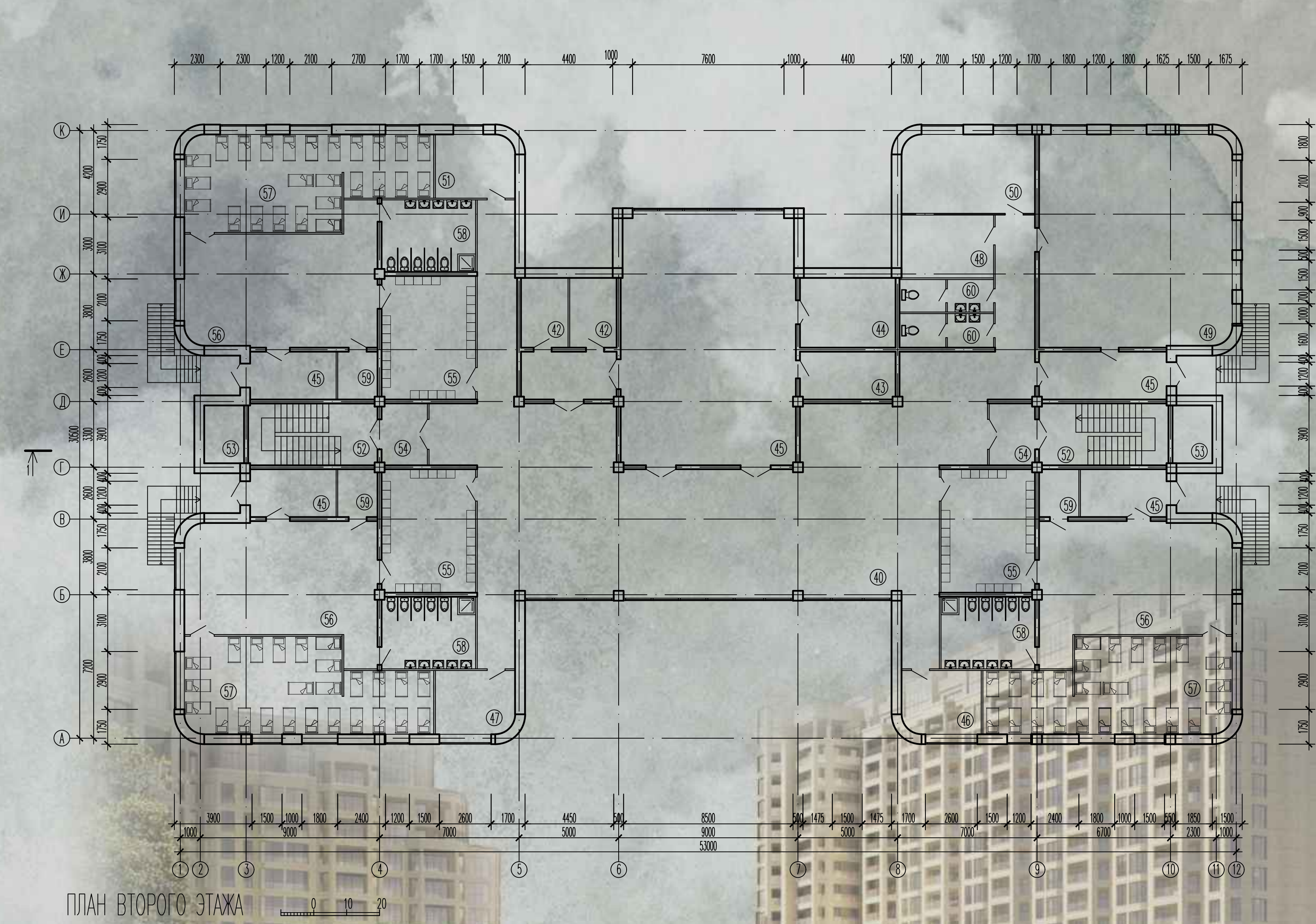
ЭКСПЛИКАЦИЯ ПОМЕЩЕНИЙ 2-ГО ЭТАЖА
